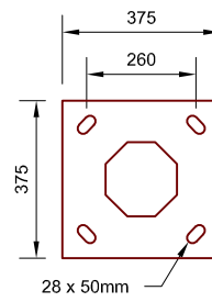
375x375x20 Flange 1 off (SCALE 1:20)
