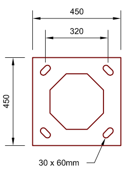
450x450x20 Flange 1 off (SCALE 1:20)
